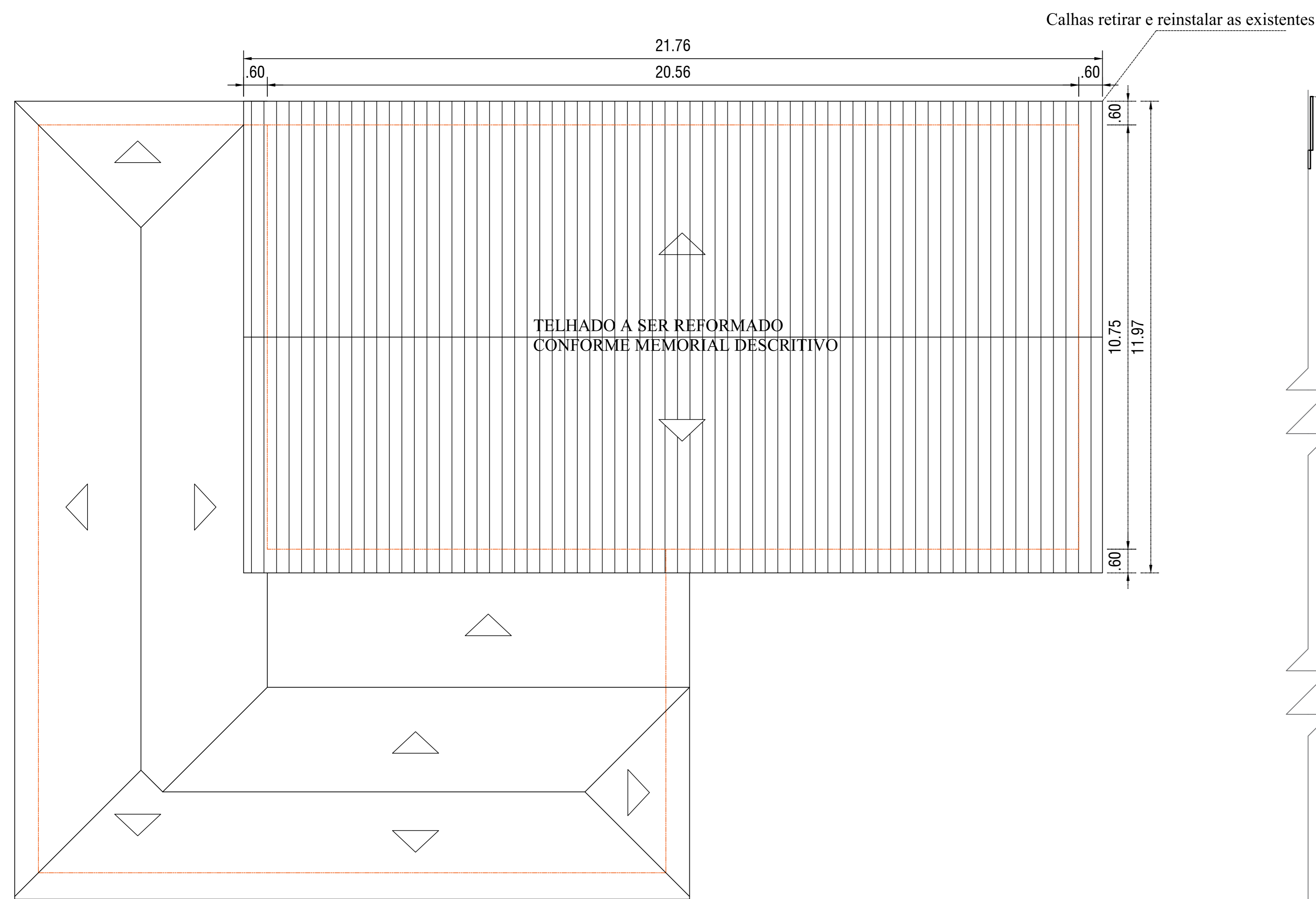
PLANTA COBERTURA AREA A REFORMAR COBERTURA: 260,21 M 2 AREA A REFORMAR BEIRAL: 39,20 M 2
