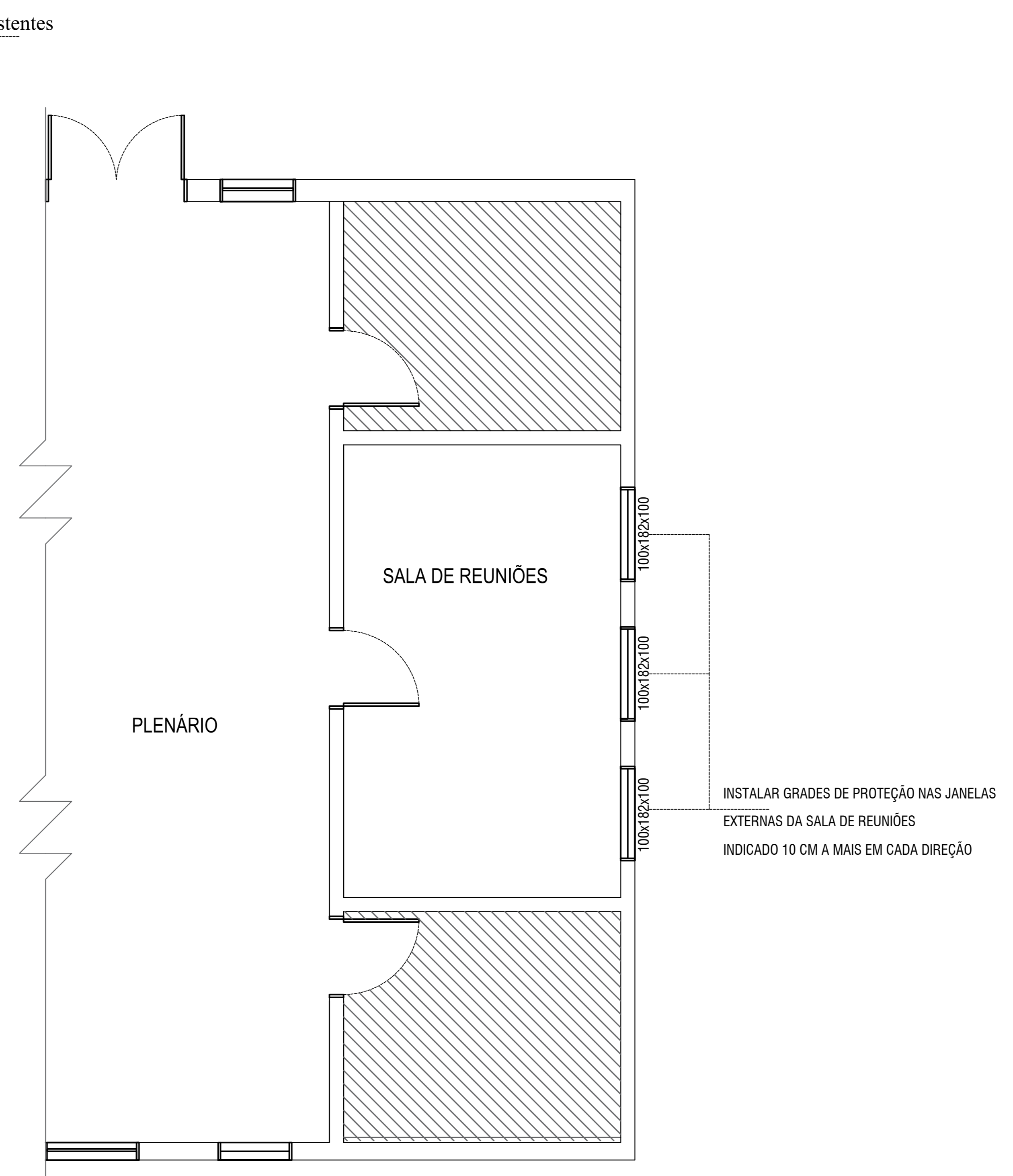
PLANTA BAIXA SALA DE REUNIÕES
