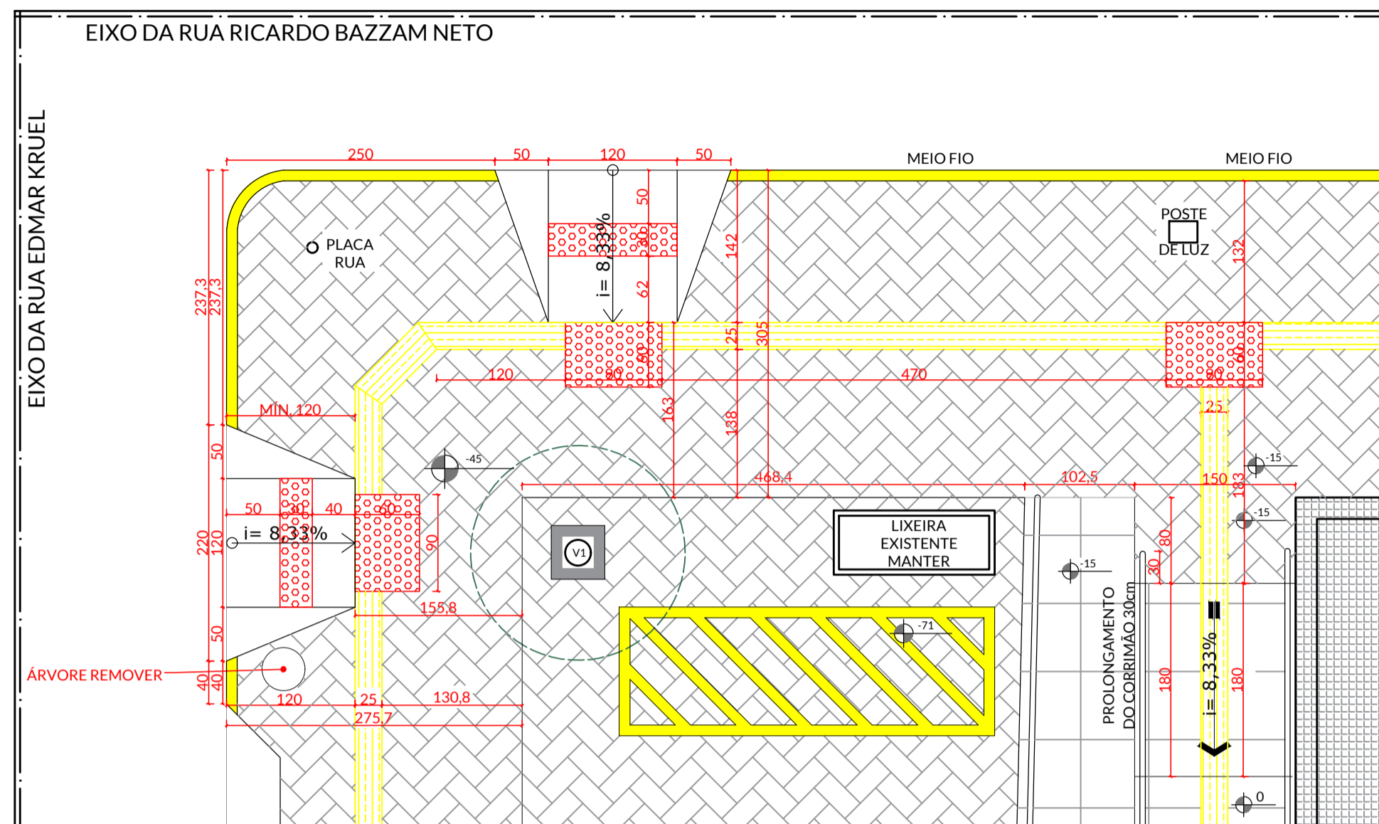
PLANTA BAIXA - DETALHE ESQUINA ESCALA: 1:50
